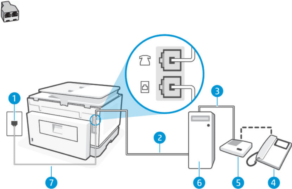
Рисунок 7-4 Параллельный разветвитель
