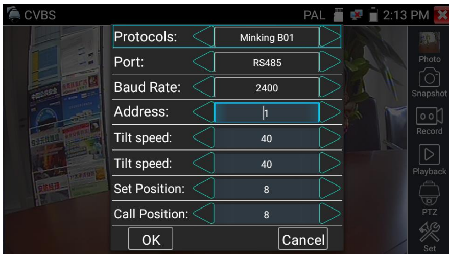
Рис.8 Настройки PTZ для RS-485
