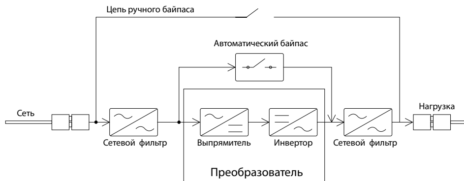
Рисунок 7. Структурная схема принципа работы стабилизатора
