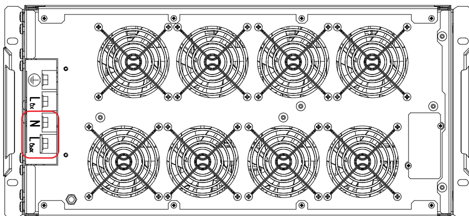
Рисунок 21. Стабилизатор Штиль IS20000RT. Выводы «N-Lвых».
