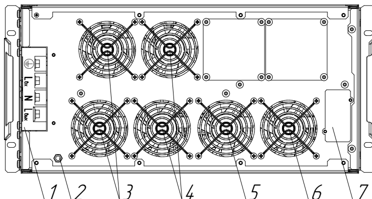
Рисунок 5. Внешний вид и компоненты задней панели стабилизаторов Штиль IS12000RT и IS15000RT
