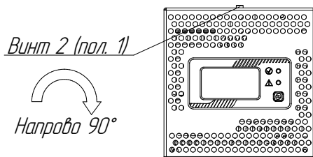
Рисунок 17а. Винт 2 в положении 1 и направление поворота поворотной части передней панели
