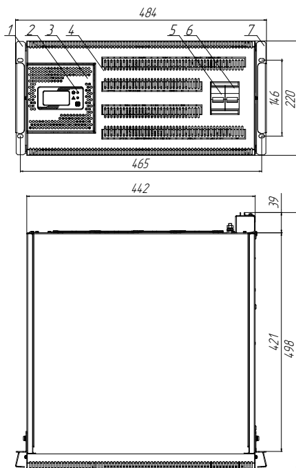
Рисунок 3а. Габаритные размеры и компоненты стабилизатора Штиль IS15000RT (горизонтальная установка)
