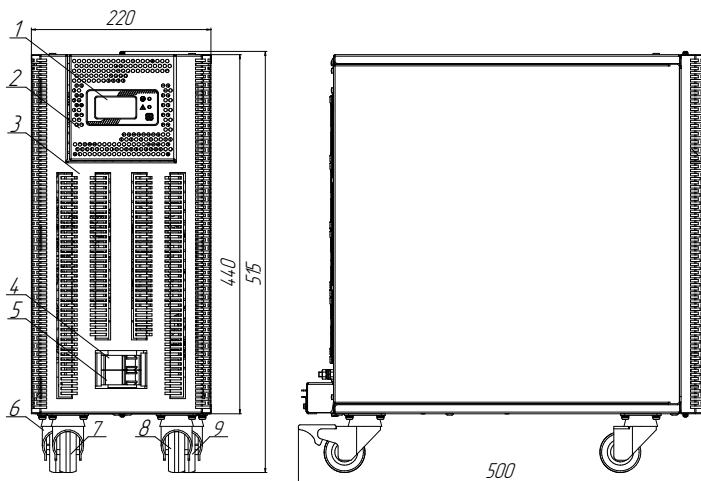
Рисунок 2б. Габаритные размеры и компоненты стабилизатора Штиль IS12000RT (вертикальная напольная установка)
