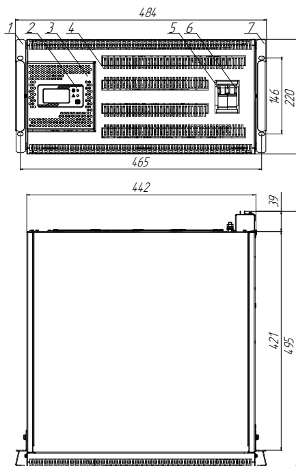
Рисунок 2а. Габаритные размеры и компоненты стабилизатора Штиль IS12000RT (горизонтальная установка)
