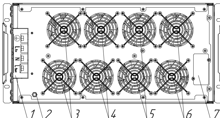
Рисунок 6. Внешний вид и компоненты задней панели стабилизатора Штиль IS20000RT
