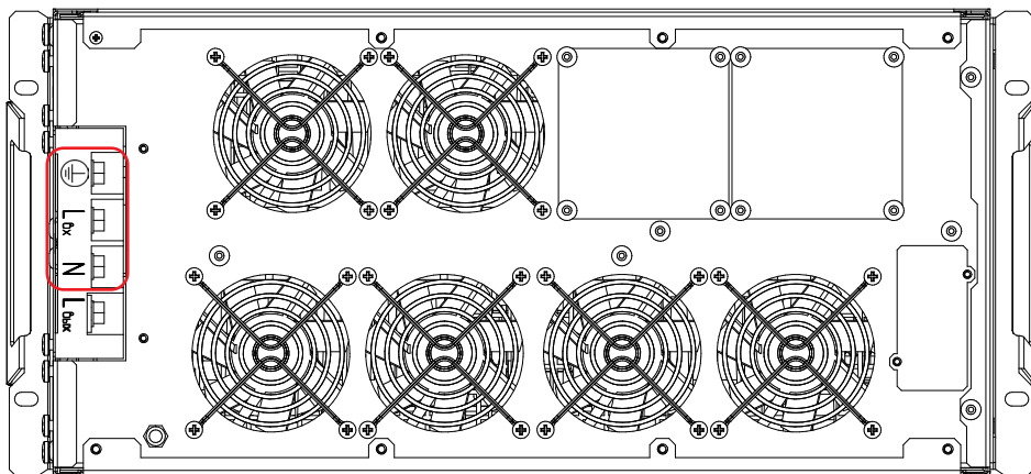
Рисунок 18. Стабилизаторы Штиль IS12000RT и IS15000RT. Выводы « \perp -Lvx-N».
