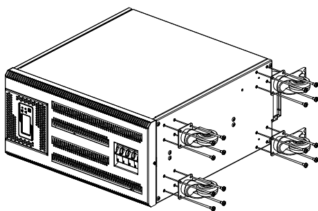
Рисунок 13. Крепление поворотных колёс к стабилизатору IS20000RT 3
