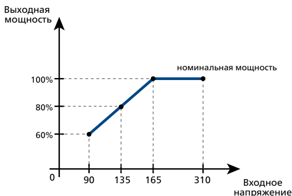
Рисунок 12. Зависимость выходной мощности от входного напряжения
