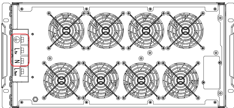
Рисунок 19. Стабилизатор Штиль IS20000RT. Выводы « \perp -Lvx-N».
