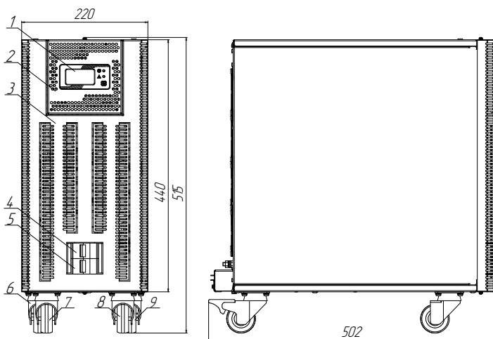
Рисунок 3б. Габаритные размеры и компоненты стабилизатора Штиль IS15000RT (вертикальная напольная установка)
