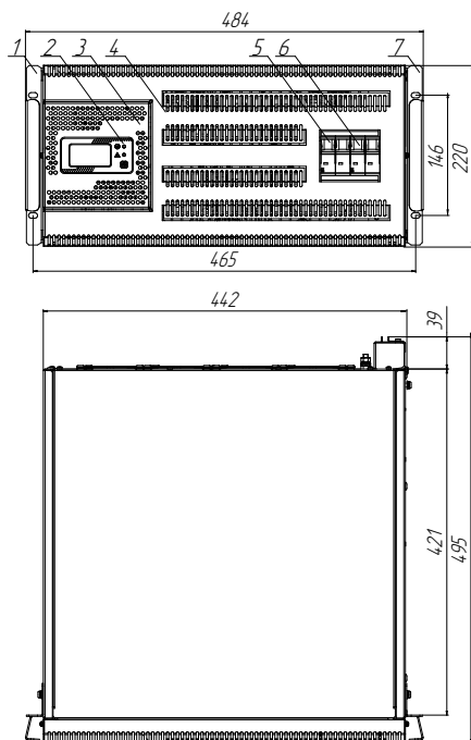
Рисунок 4а. Габаритные размеры и компоненты стабилизатора Штиль IS20000RT (горизонтальная установка)
