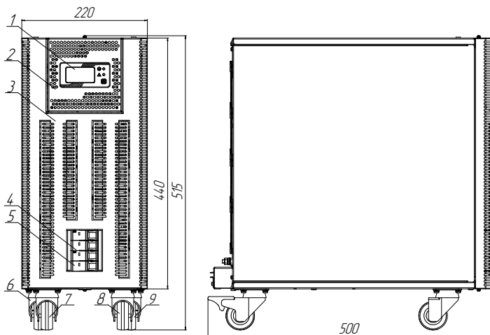
Рисунок 4б. Габаритные размеры и компоненты стабилизатора Штиль IS20000RT (вертикальная напольная установка)
