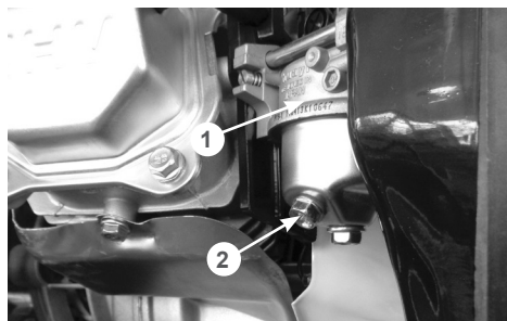
Рис. 20 Слив топлива из карбюратора
