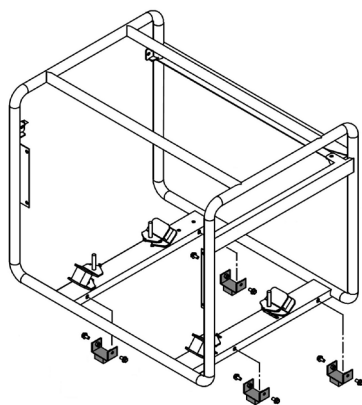
Рис. 4 Установка опор рамы
