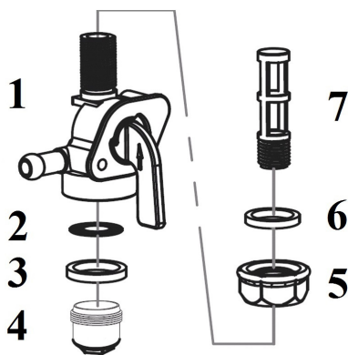
Рис. 19 Устройство топливного крана
