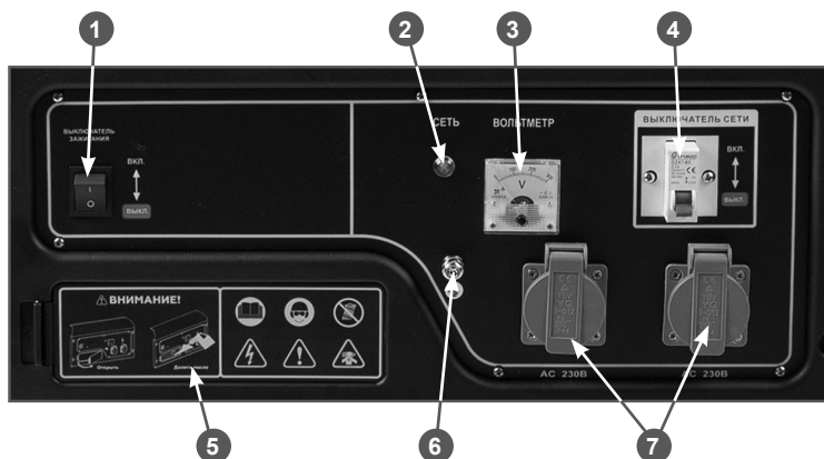
Рис. 3 Панель управления
