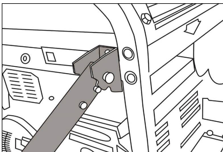
Рис. 6. Установка ручек
