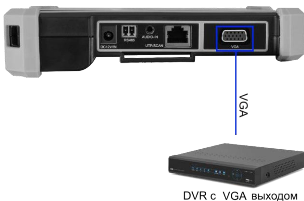
Рис. 11 Подключение VGA устройств к тестеру.
