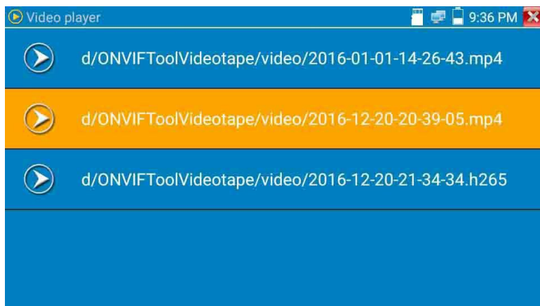
Рис. 40 Меню видеоплеера
