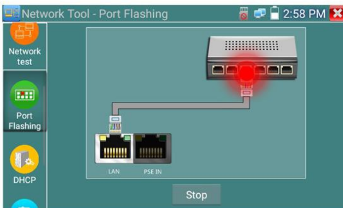
Рис. 94 Интерфейс инструмента «Определение порта» (Port Flashing)
