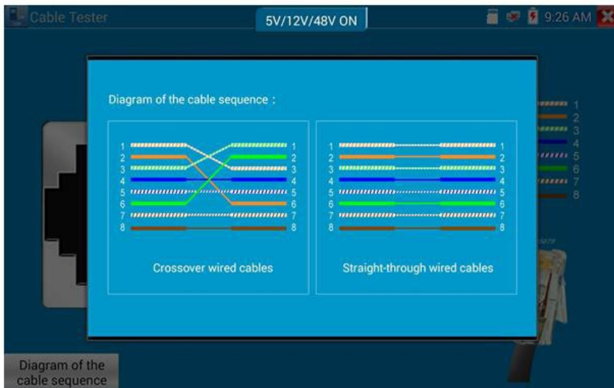
Рис. 101 Диаграммы обжимки разными методами кабеля «витой пары»
