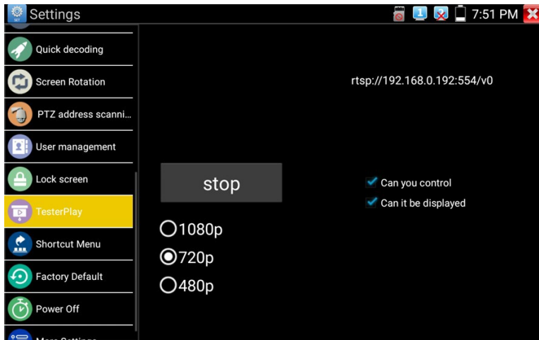
Рис. 17 Приложение TesterPlay
