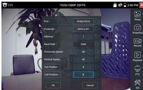
Рис.79 Управление PTZ CVI видеокамерой по интерфейсу RS232/485
