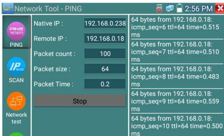
Рис. 88 Интерфейс инструмента «PING тест»
