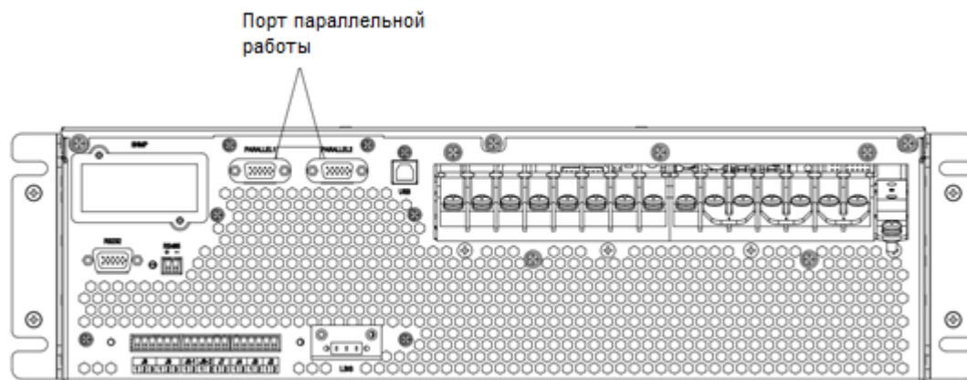
Рисунок 41. Расположение платы параллельной работы
