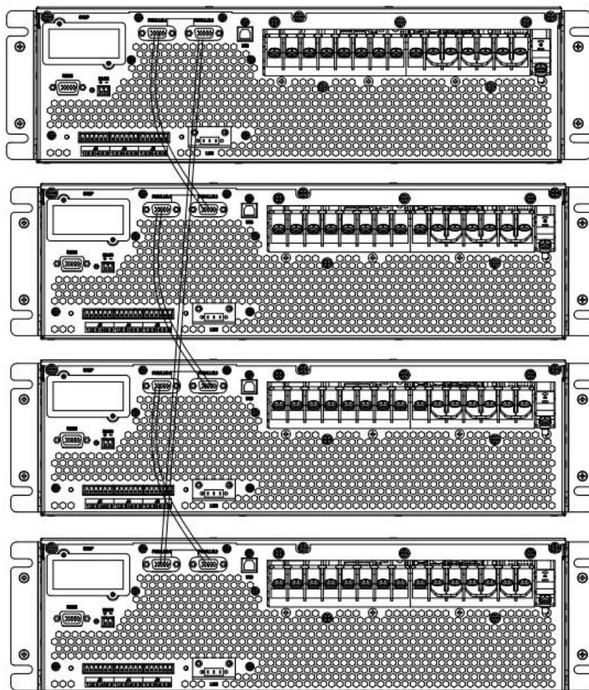
Рисунок 42. Схема соединения
