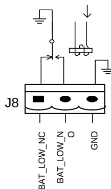
Рисунок 17. Сухой контакт сигнала о низком заряде АКБ
