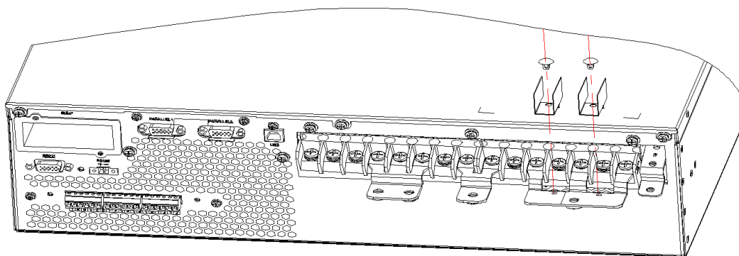
Рисунок 24. Установка изоляционной планки
