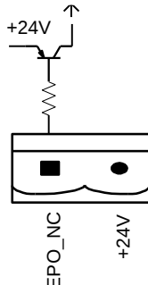
Рисунок 15. Контакты аварийного отключения
