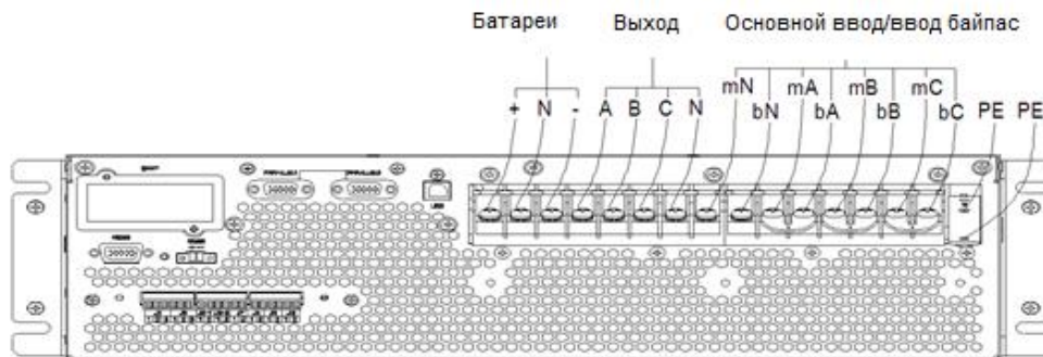
Рисунок 18. 3 фазы вход/3 фазы выход (общий ввод)
