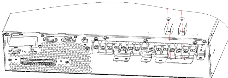
Рисунок 21. Установка изоляционной планки
