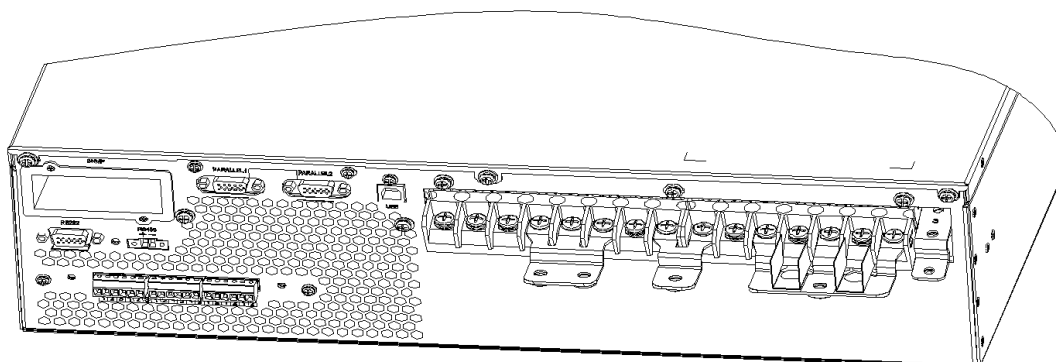
Рисунок 25. Фиксация изоляционной планки
