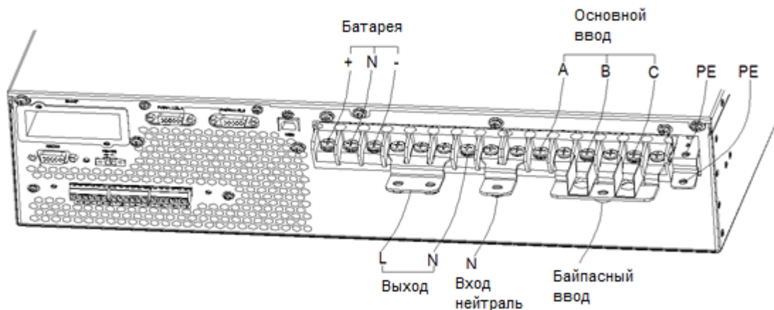
Рисунок 23. Подключение 3 фазы вход/1 фаза выход (при питании ИБП от двух вводов)
