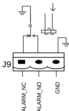
Рисунок 18. Сигнализация об аварии (общий)
