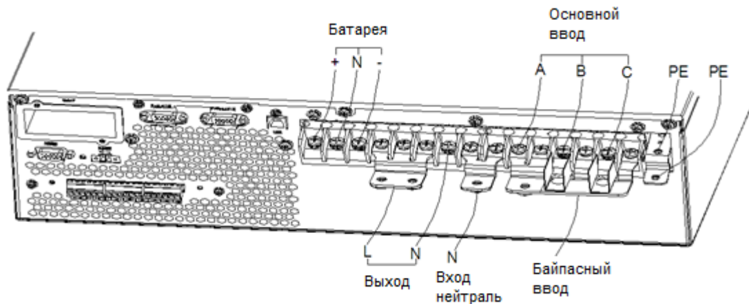
Рисунок 21. Подключение 3 фазы вход/1 фаза выход (при питании ИБП от одного общего ввода)
