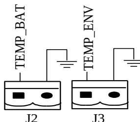
Рисунок 14. Контакты J2 и J3 для определения температуры
