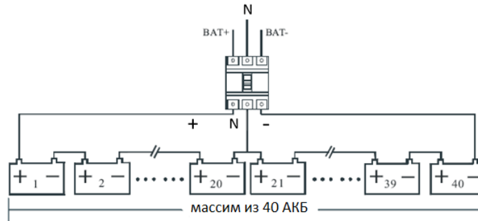
Рисунок 11. Схема подключения батарей
