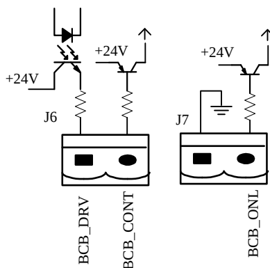
Рисунок 16. Контроль ВСВ (управление автоматическим выключателем АКБ)
