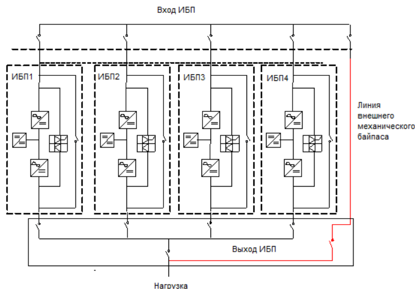
Рисунок 40. Схема параллельной системы
