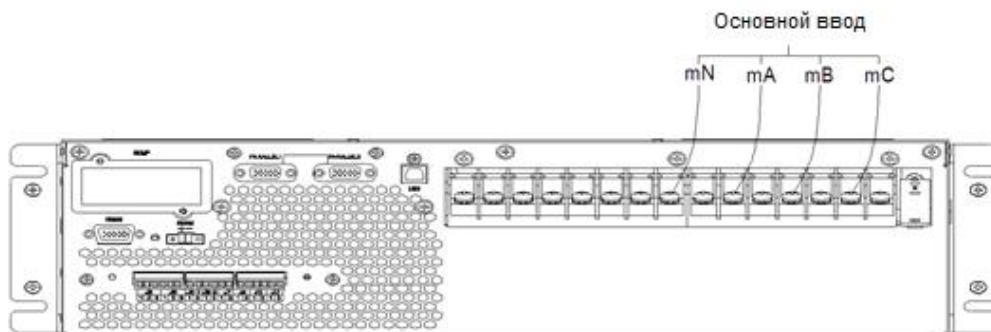
Рисунок 20. Подключение основного ввода
