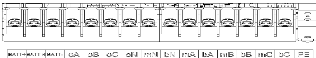
Рисунок 12. Терминалы для подключения кабелей
