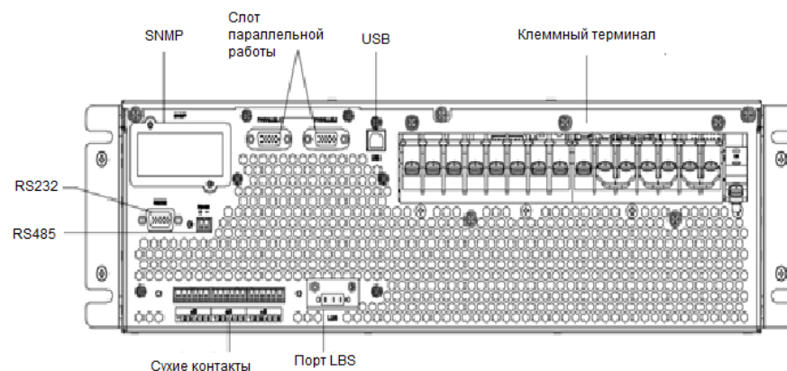
Рисунок 1. (б) Внешний вид ИБП 10-15 КВА (вид сзади)
