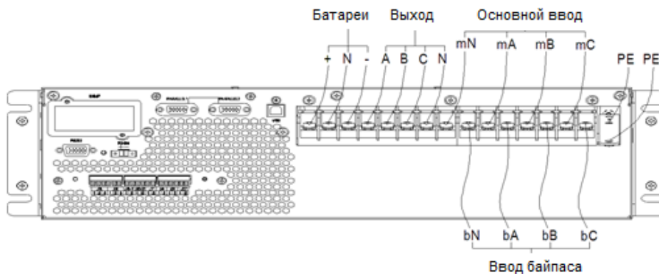
Рисунок 19. 3 фазы вход/3 фазы выход (от двух вводов)
