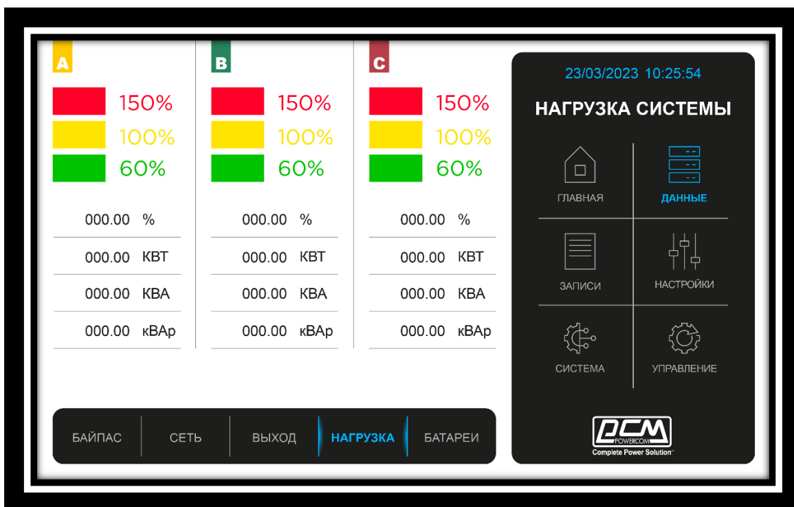
Рисунок 31. Подменю раздела «Данные»
