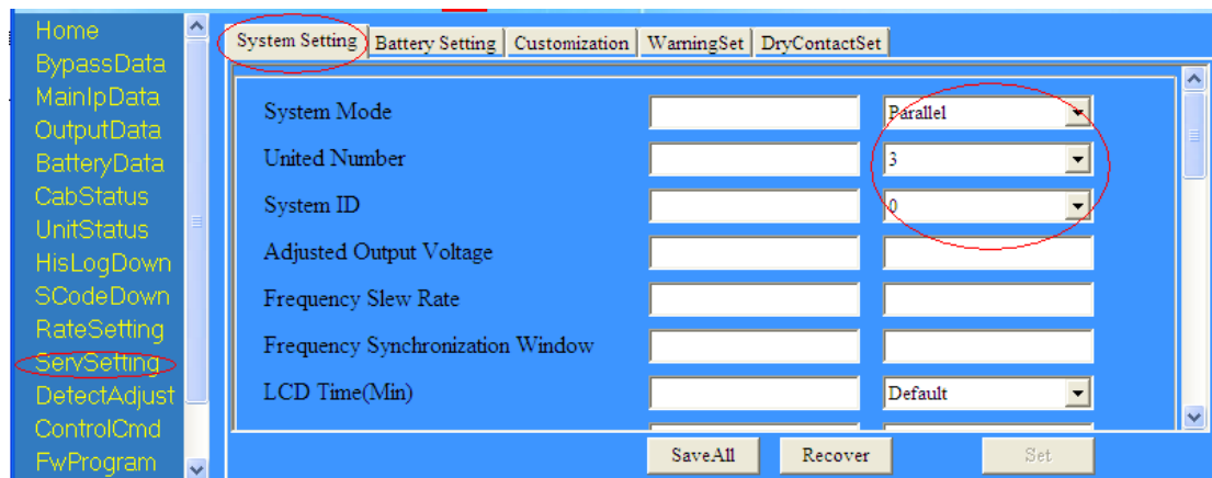
Рисунок 43. Настройка параллельной системы
