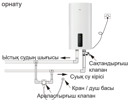
1-сурет. Орнату сұлбасы- көлденең орнату
