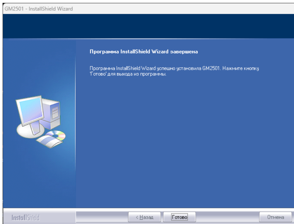
Рисунок 23 – Завершение установки
