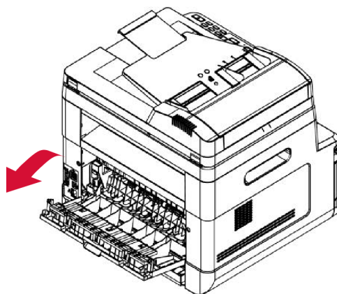
Рисунок 49 – Открытие задней крышки
