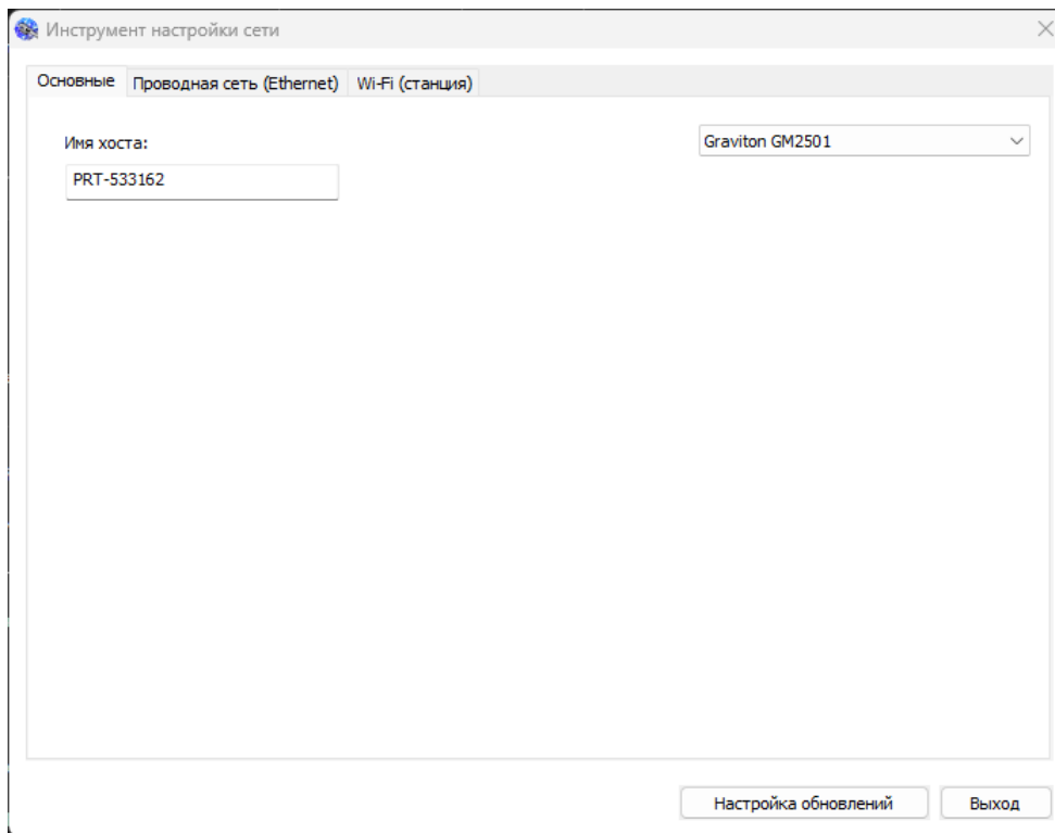
Рисунок 28 – Вкладка «Основные»
