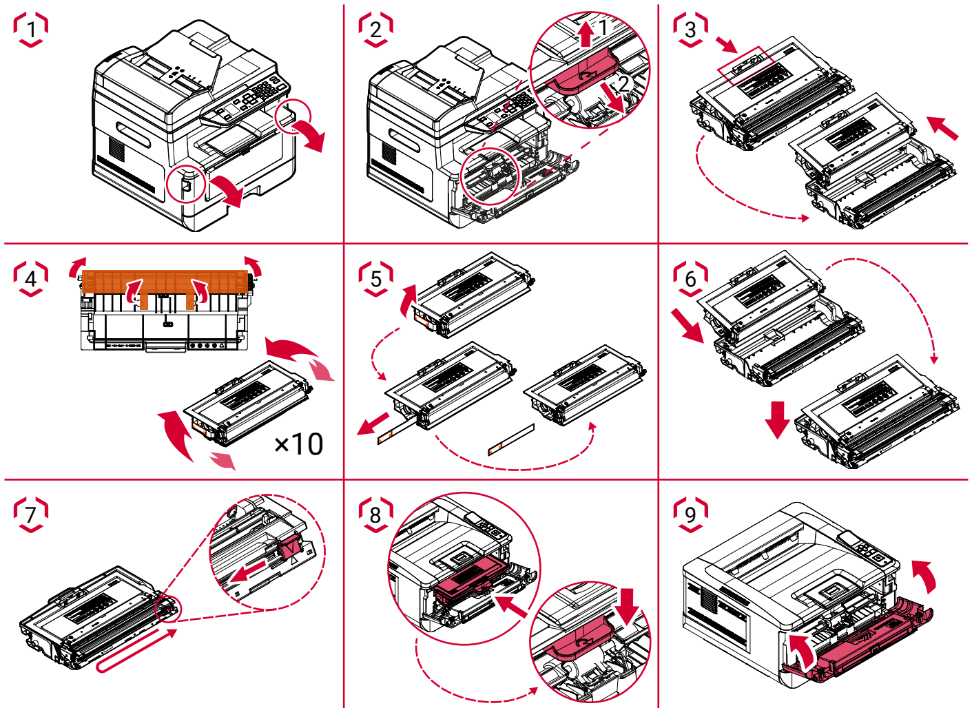
Рисунок 43 – Замена картриджа
