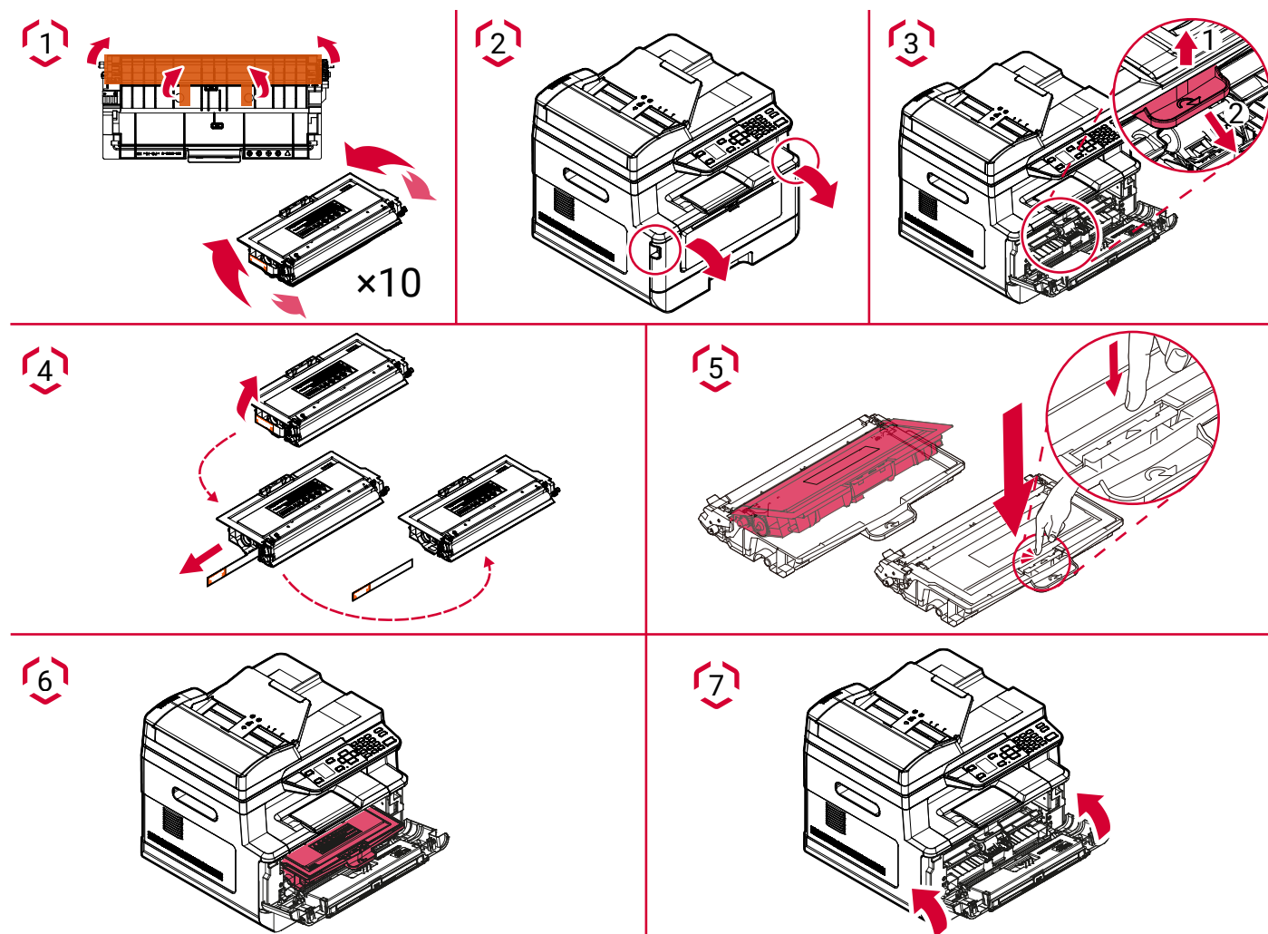
Рисунок 9 – Установка картриджа
