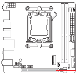
PCI_E1: PCIe 5.0 x16 (от процессора)
