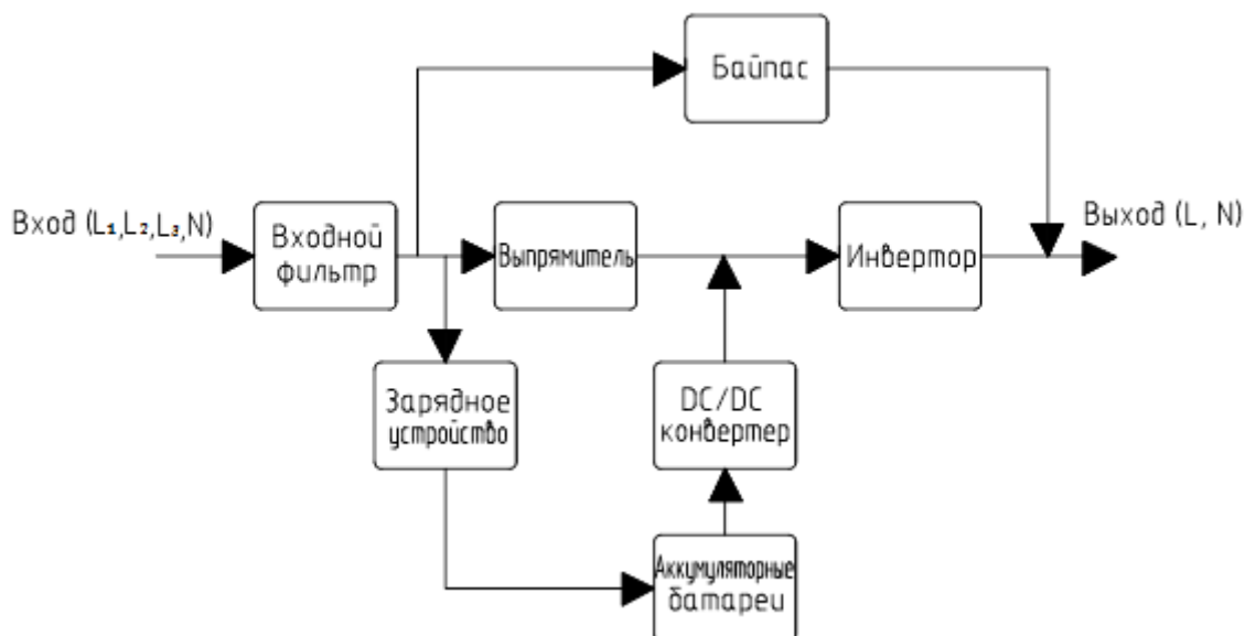
Рисунок 1.5 – Функциональная схема работы изделия
