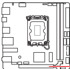
PCI_E1: PCIe 5.0 x16 (от процессора)
