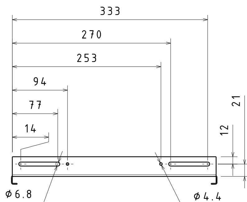
Вид слева Масштаб: 1:4
