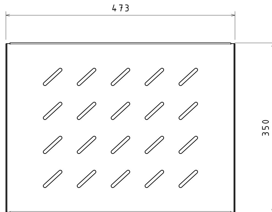
Вид сверху Масштаб: 1:4
