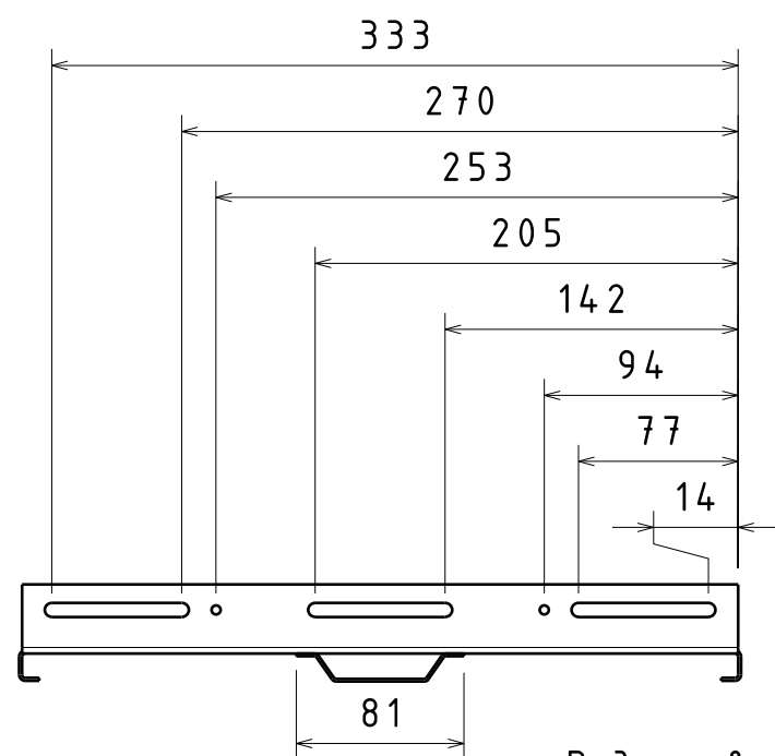
Вид справа Масштаб: 1:4
