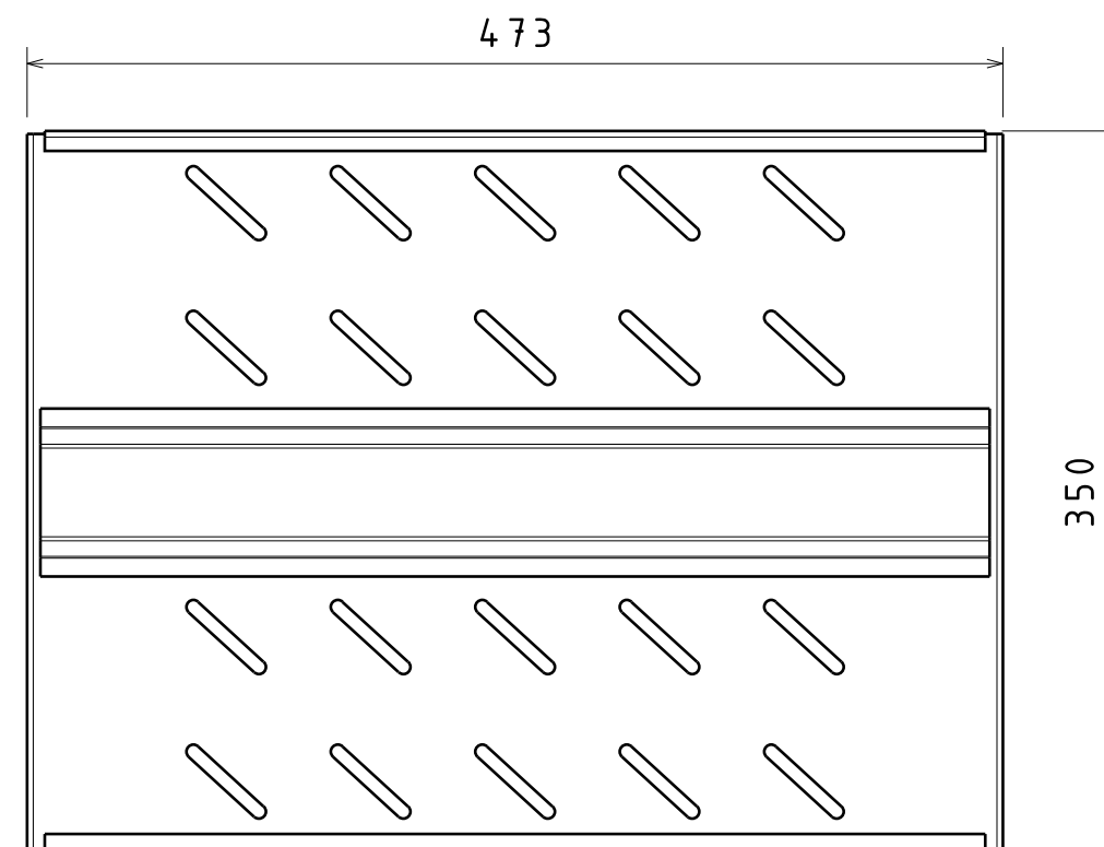
Вид снизу Масштаб: 1:4
