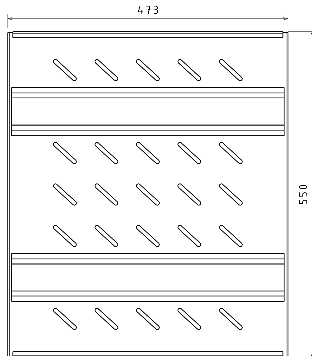
Вид снизу Масштаб: 1:4
