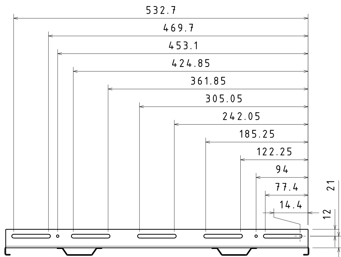
Вид справа Масштаб: 1:4
