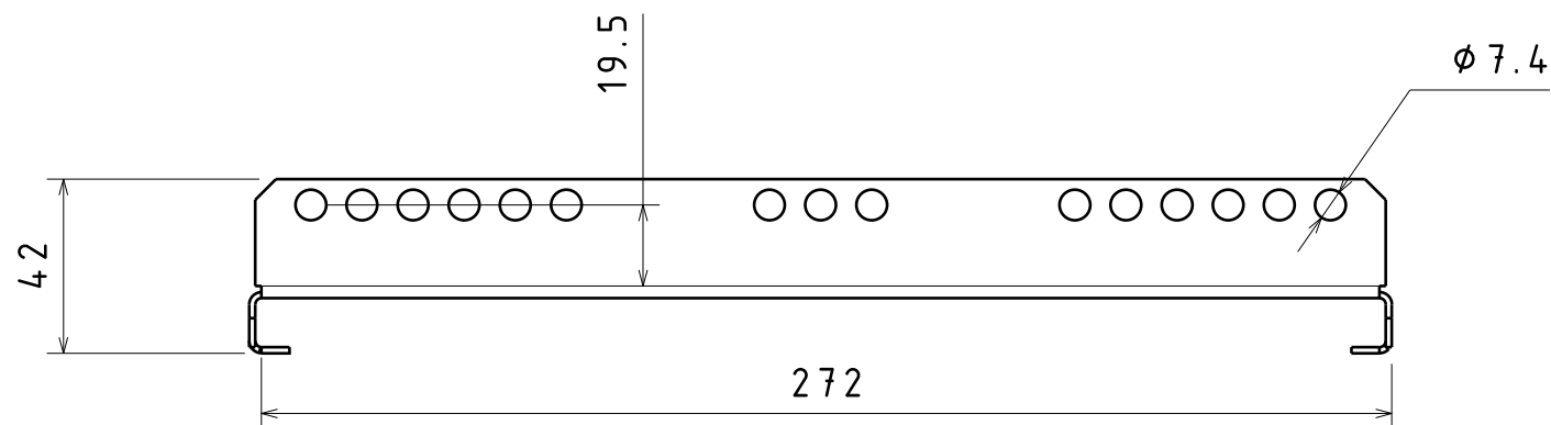
Вид справа Масштаб: 1:2
