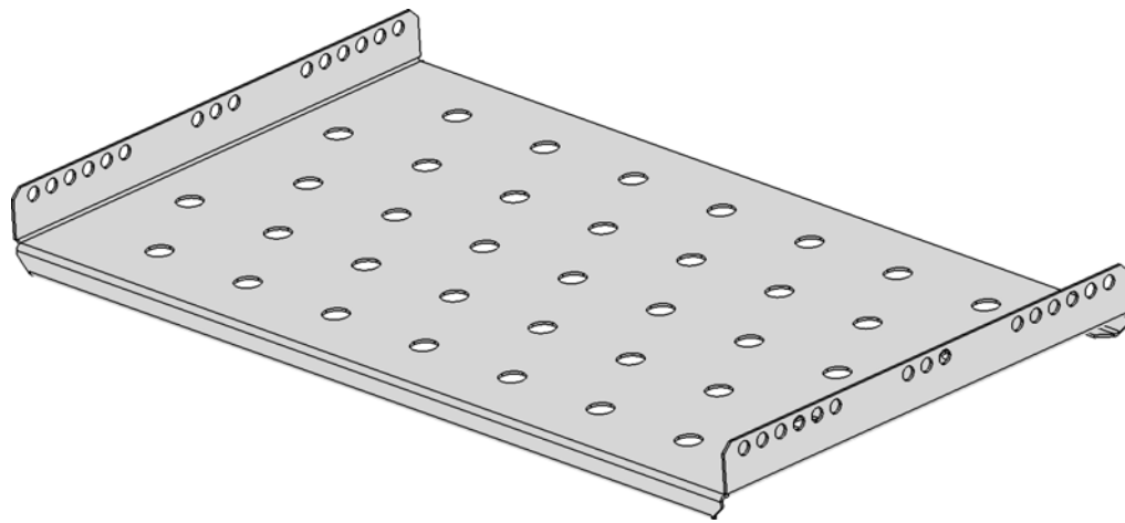
Вид изометрия Масштаб: 1:4
