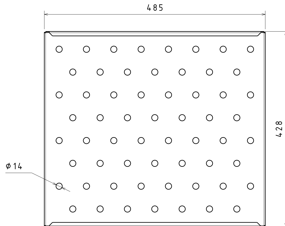
Вид снизу Масштаб: 1:4
