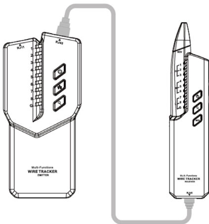
Рисунок 11 – Проверка патч-корда
