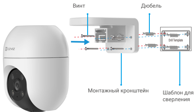
Рисунок 2. Монтаж на стену
