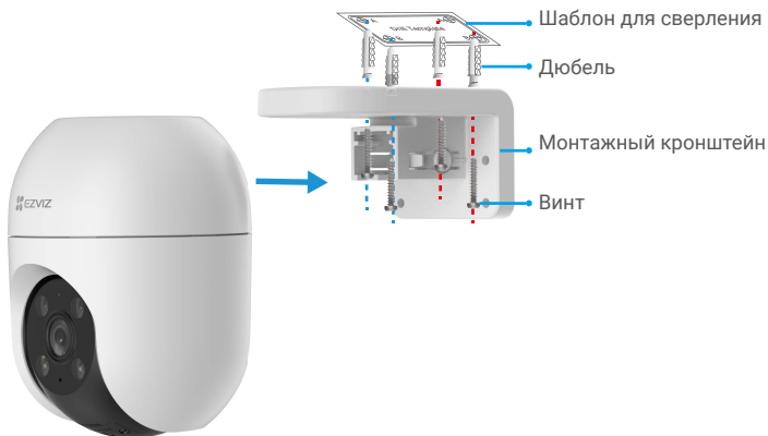
Рисунок 1. Монтаж на потолок
