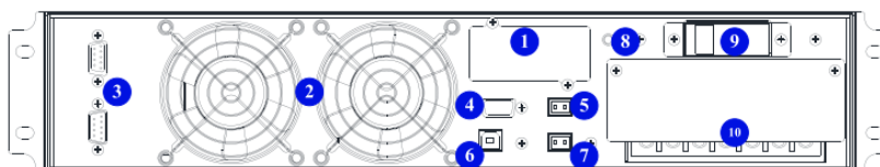
Рисунок 7-2. Задняя панель
