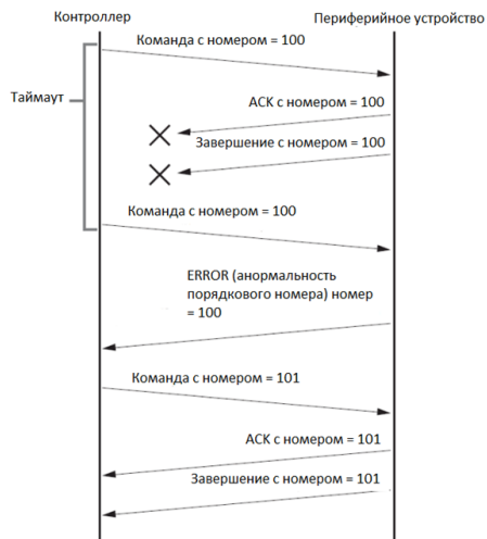
Схема последовательности операций при потере возвращаемого сообщения
