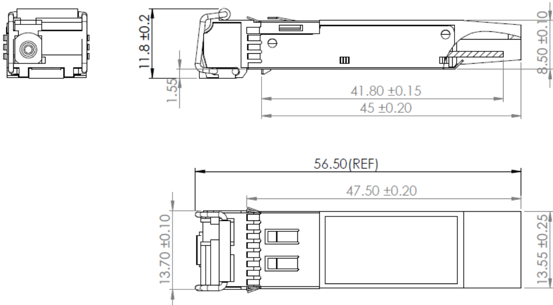
LAN-WDM+12/13-20-SM, LAN-WDM+13/12-20-SM
