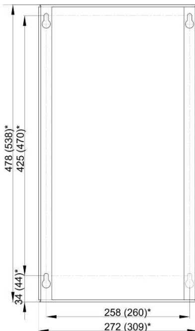
Рисунок 3 – Крепление изделия на стену (размеры со звёздочкой* — для ST-20000 LED, ST-30000 LED)
