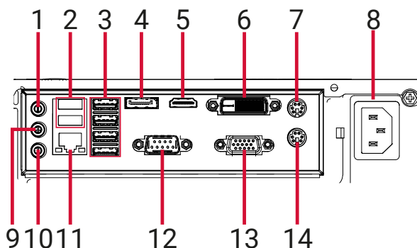
Рисунок 2 – Задняя панель
