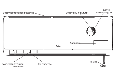
Рис. 1. Внутренний блок*
