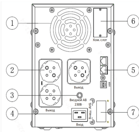
Рисунок 7-2. Вид сзади
