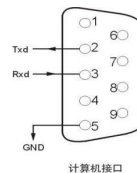
计算机接口
