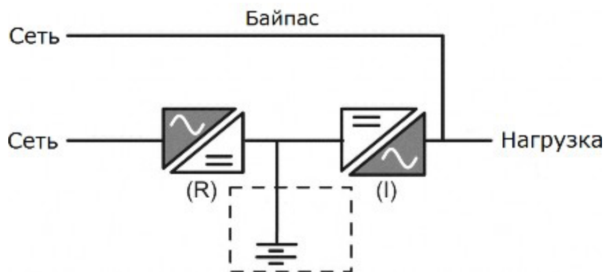
Рис. 2. Блок-схема
