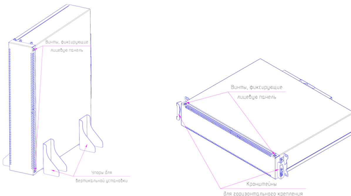
а) вертикальная установка
