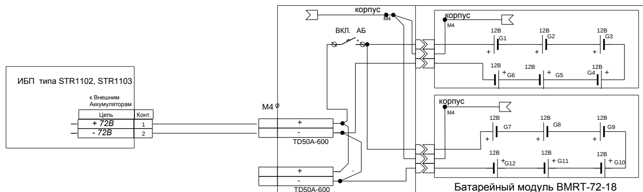
Рисунок 3 - Схема электрическая соединений
