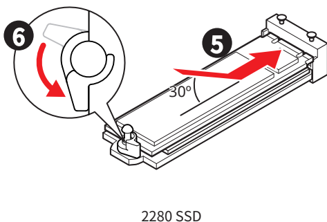
2280 SSD
