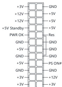
ATX_PWR
