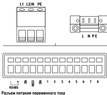
Рис. 2.1 Интерфейс подключения (данные о порте энергоснабжения содержатся в указаниях на заводской табличке с паспортными данными)
