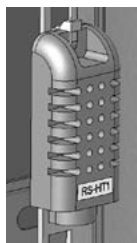
Рисунок 12. Датчик температуры и влажности цифровой RS-HT1
