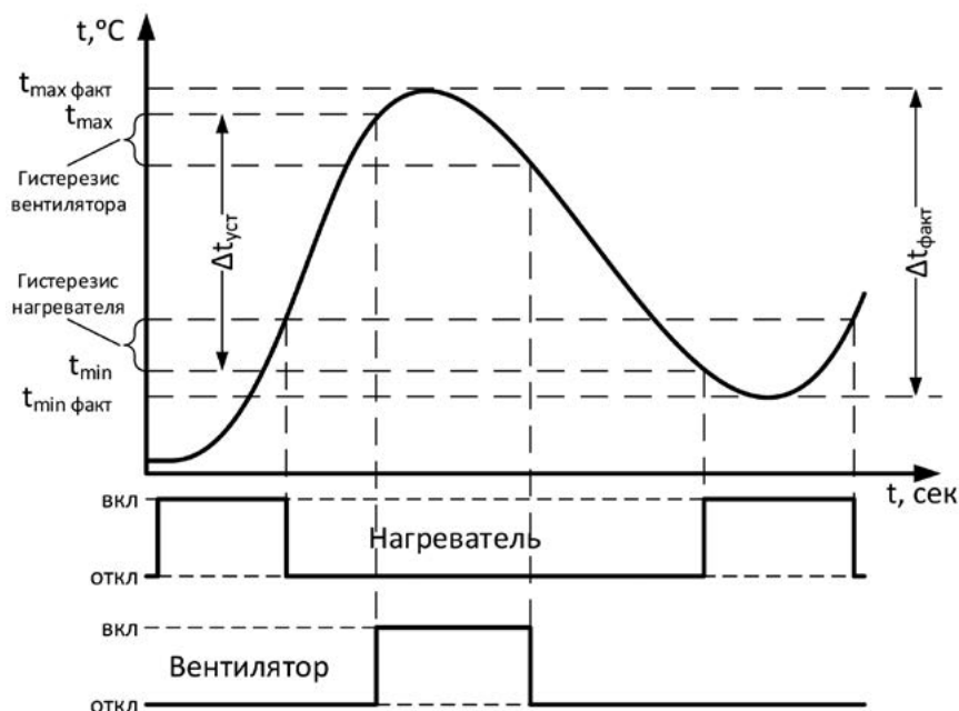
Рис. 3. Пороговое регулирование температуры
