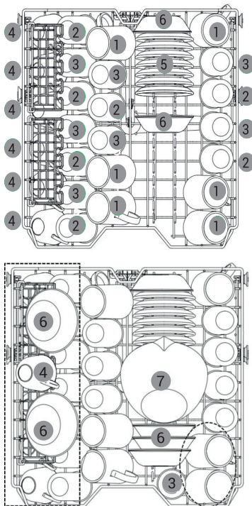
Схема загрузки 15 наборов (вариант 2)
