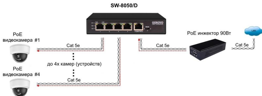
Рис.4 Типовая схема подключения коммутатора SW-8050/D в режиме получения питания от PoE инжектора
