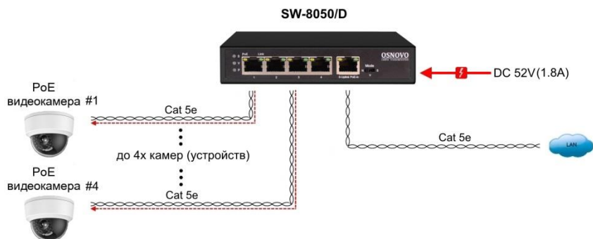
Рис.5 Схема подключения коммутатора SW-8050/D в режиме питания от БП и передачи PoE к окончательным устройствам
