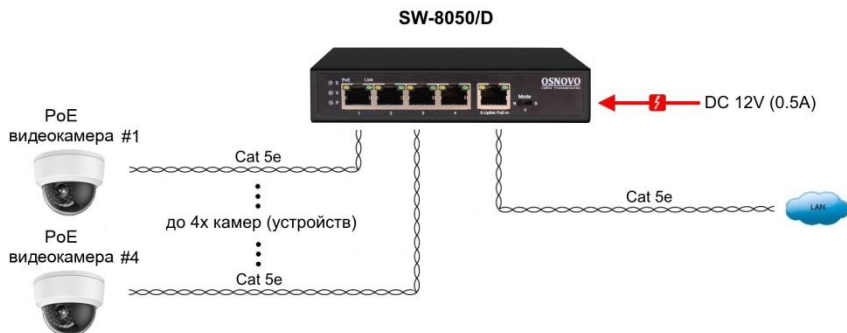
Рис.6 Схема подключения коммутатора SW-8050/D в режиме питания от БП (только передача данных, без использования PoE)
